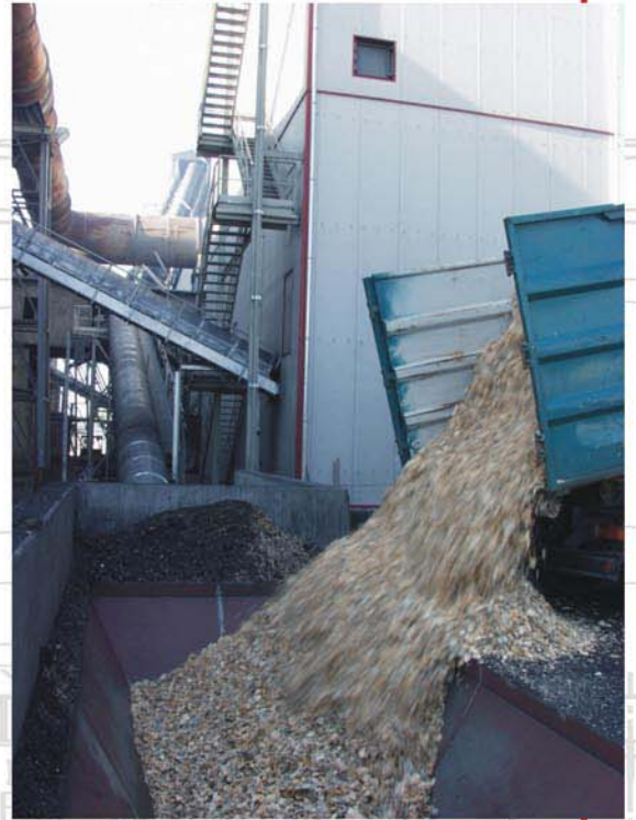
Carico di chips di legno in tramoggia di ricezione per insilaggio automatico
